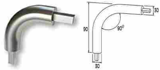
UNIÓN ENTRE RAILES EN 90º Connector 90° for F50-307 guide / Code 4243 / Pack. 10 /pcs.
