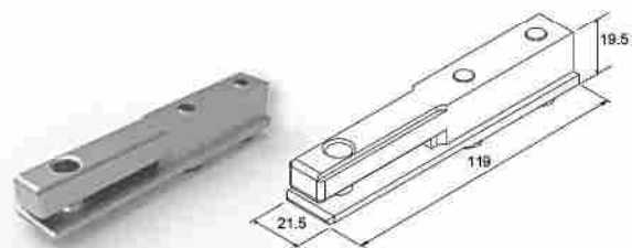
CALIBRE DE LOS AGUJEROS PARA F50-319 Holes calibre for F50-319 / Code 4971 / Pack. 1 /pc.
