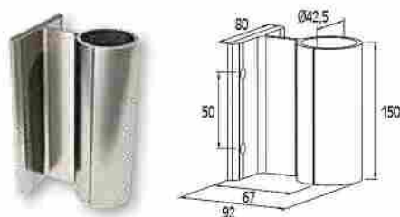
PIE DE SOPORTE EXTERIOR 15 cm PARA COLUMNA F50-100
