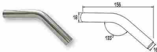
VARILLA CONECTORÁ F16 EN 90° Connector 135° for profile Ø16
