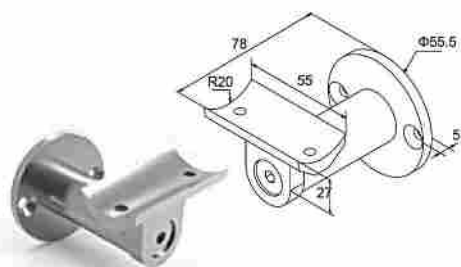
SOPORTE DE PARED A PASAMANOS DE 40MM
