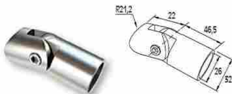
ARTICULACION COLUMNA F50-100 CON PERFIL F26 Connector for F50-100 column with profile Ø26
