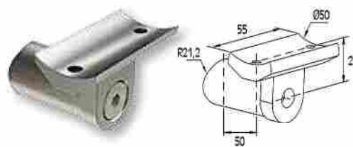
SOPORTE COLUMNA EXTERNO F50-100 Y F-50-200
