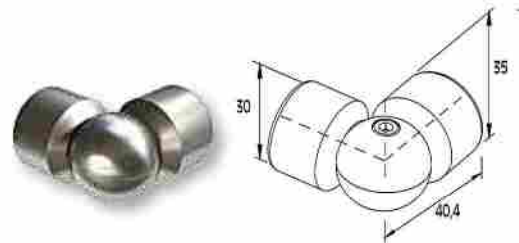
ARTICULACION PARA PASAMANOS EN ESQUINA F50-307 Adjustable corner connector for F50-307 guide
