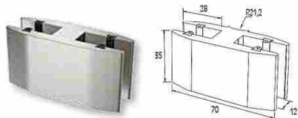
PINZA DOBLE PARA CRISTAL DE 8-10mm PARA COLUMNA F50-103 Double glass support 8-10 mm for F50-103 column
