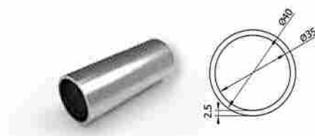
PERFIL PASAMANOS F40 Handrail Ø40
