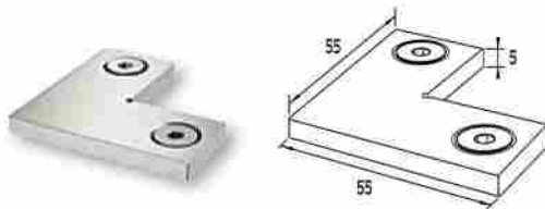
UNION DE PASAMANOS EN 90º PARA F50-201 Connector 90° for F50-201 handrail / Code 4250 / Pack. 50 /pcs.
