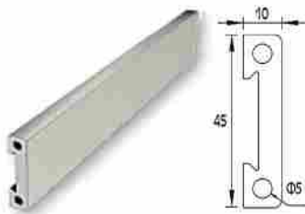
PERFIL EMBELLECEDOR Blade column
