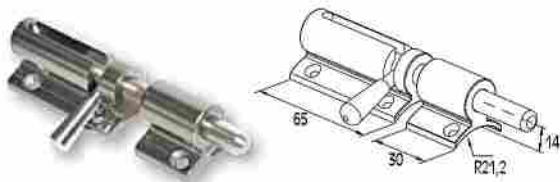
CERROJO PARA LA COLUMNA F50-100 Bolt for F50-100 column
