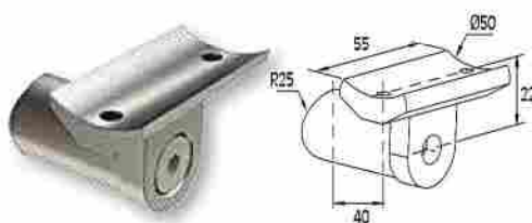
SUJECCIÓN EXTERNA A PASAMANOS External Support for F50-200 handrail to F50-101 column
