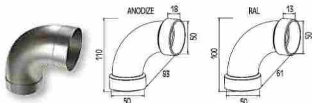
UNIÓN ESQUINA PASAMANOS 90° Connector 90° for handrail Ø50
