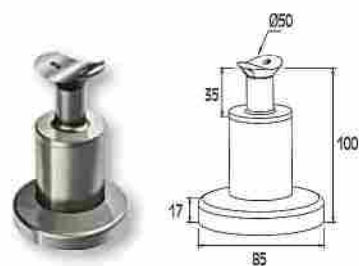
SOPORTE DE 8.5 CM PASAMANOS A MURO
