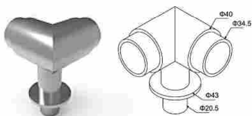
CONECTOR DE PASAMANOS DE 40MM
