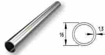
PERFIL F-16 X 1,3 MM DE GROSOR Profile Ø16X1,3 / Code F50-300 / Weight 162 gr/m
