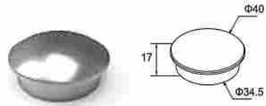
TAPA PARA PASAMANOS DE 40MM End cap for handrail Ø40
