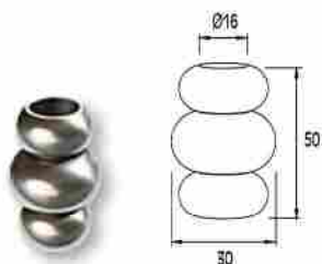
DECORACIÓN PERFIL PARA ESCALERA F-16 Glass rosette for profile Ø16 / Code 4618 / Pack. 50 /pcs.
