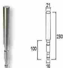
SUJECCIÓN COLUMNA F50-100 & F50-101 AL SUELO Infloor support for Ø42 columns
