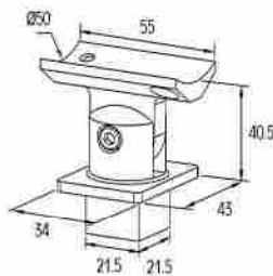
UNION COLUMNA CON PASAMANOS F50-200 F50-200 Railtop support stairs
