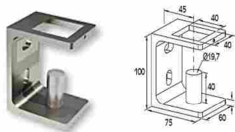
SOPORTE EXTERIOR PARA COLUMNA F50-102 External support for F50-102 column
