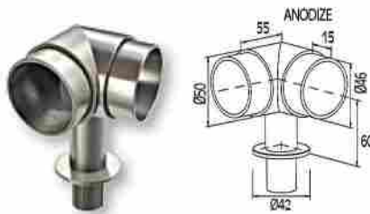
UNIÓN PASAMANOS EN 90° Ø50 Railtop corner Connector 90° for handrail Ø50
