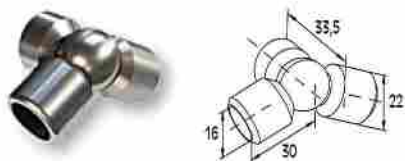
UNIÓN EN ESQUINA DE PERFIL DE 16 A COLUMNA F50-102 Adjustable corner connector for profile Ø16
