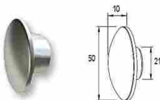
TAPA COLUMNA F50-101 End cap for F50-101 column
