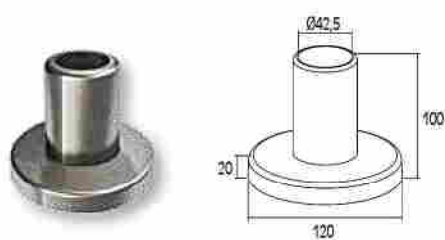
PIE DE SUJECCIÓN DE 12 CM. REFORZADO PARA COLUMNA F50-100
