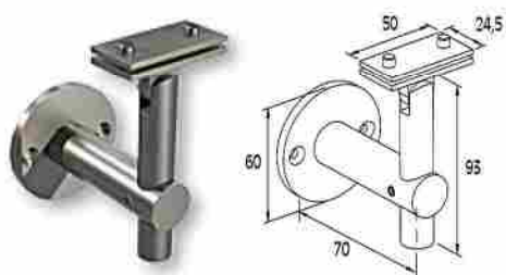
DECORACIÓN PERFIL PARA ESCALERA F-16 F50-201 Railtop wall support / Code F85-452 / Pack. 40 /pcs.
