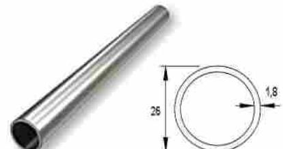
PERFIL Ø26mm inox Profile Ø26x1,8 / Code F50-304 / Weight 370 gr/m
