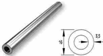
PERFIL F-16 X 3,5 MM DE GROSOR Profile Ø16X1,3 / Code F50-301 / Weight 370 gr/m
