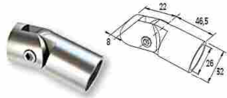
UNIÓN DE F50-102 CON PERFIL DE 26 MM Connector for F50-102 column with profile Ø26 / Code 4349 / Pack. 20 /pcs.
