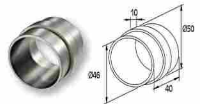
UNIÓN DE PASAMANOS CON PASAMANOS (INTERIOR)
