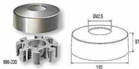
PIE DE SUJECION PARA COLUMNA F50-100
