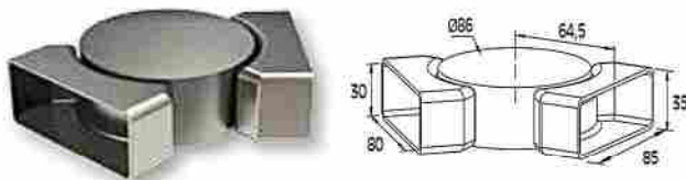
UNIÓN EN ESQUINA DE PASAMANOS F50-201, F50-203 Adjustable corner connector for F50-201/203 railtop
