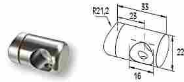
UNIÓN COLUMNA F50-100 PARA PERFIL F16 Connector for F50-100 column with guide Ø16
