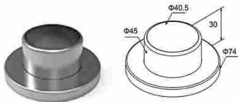
SOPORTE PARA COLUMNA REDONDA DE 40MM Wall cover for handrail Ø40
