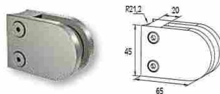
PINZA DE SUJECCION CRISTAL 8-10 MM 45 X 65
