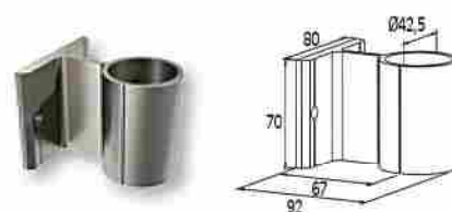
SUJECCIÓN COLUMNA A PARED F50-100 External support for Ø42 column
