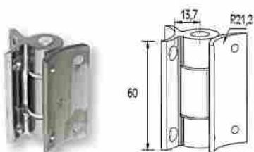
VISAGRA PARA LA COLUMNA F50-100 Hinge for F50-100 column
