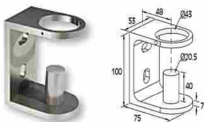
SOPORTE EXTERIOR PARA COLUMNA F50-100 External support for F50-100/103 columns
