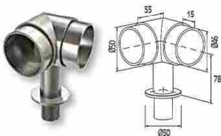
ARTICULACIÓN DE PASAMANOS EN 90° PARA F50-101
