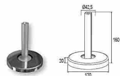
PIE DE SUJECCIÓN DE 12CM PARA COLUMNA F50-100
