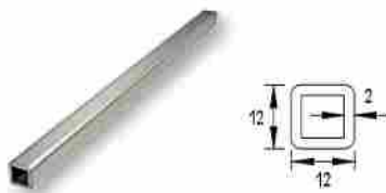
COLUMNA CUADRADA DE 12 X 12 X 2mm Column 12x12x2
