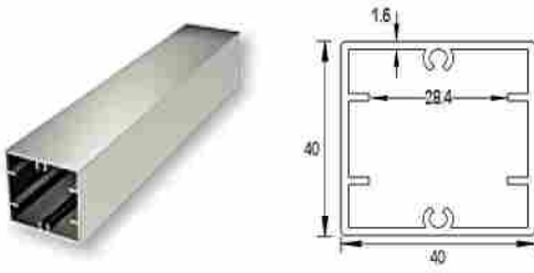
PERFIL CUADRADO 40 X 40 Support column 40x40
