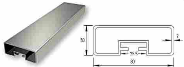
PASAMANOS 30 X 80 Handrail 30x80
