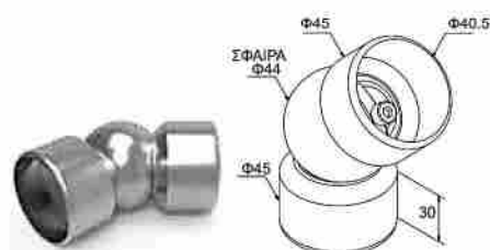
CONECTOR PARA PASAMANOS DE 40MM
