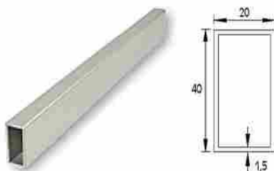
PERFIL 40 X 20 40x20 Profile
