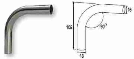
VARILLA CONECTORÁ F16 EN 90° Connector 90° for profile Ø16
