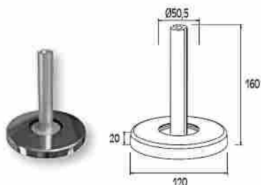
PIE DE SUJECCIÓN DE 12 CM. PARA COLUMNA F50-101
