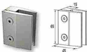
PINZA PLANA PARA CRISTAL 8-10mm COLUMNA F50-102, F50-106
