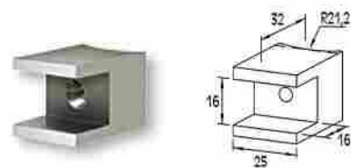
UNIÓN COLUMNA F50-100 CON PERFIL F50-302 (SUJECION EXTERIOR)
