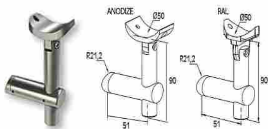
SUJECCIÓN PASAMANOS F-50 COLUMNA External support for handrail Ø50-column Ø42
