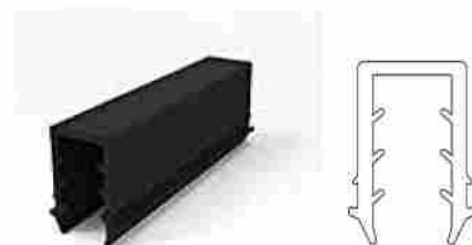
GOMA CON FORMA DE U PARA 10.76 DE CRISTAL "U" shape gasket for 10.76 mm glass (5 mm-2PVB-5 mm) / Code 4910 / Pack. 40 m
