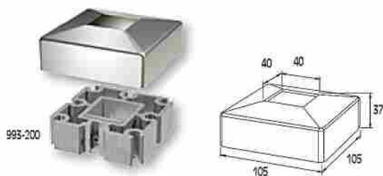
PIE DE SUJECION PARA COLUMNA F50-102, F50-106
