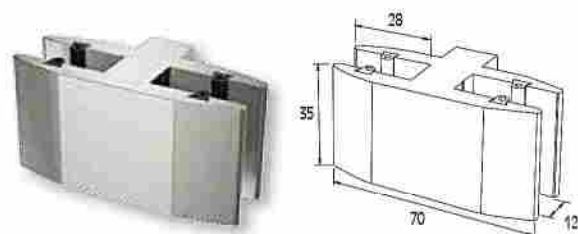
PINZA DOBLE PARA CRISTAL 8-10mm COLUMNA F50-102 Double glass support 8-10 mm for F50-102 column
