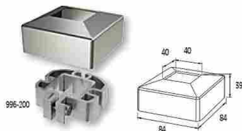
SOPORTE PARA COLUMNA DE 40 X 40
