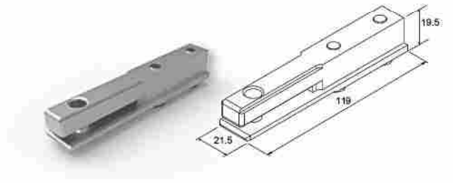
CALIBRE DE LOS AGUJEROS PARA F50-319 Holes calibre for F50-319 / Code 4971 / Pack. 1 /pc.
