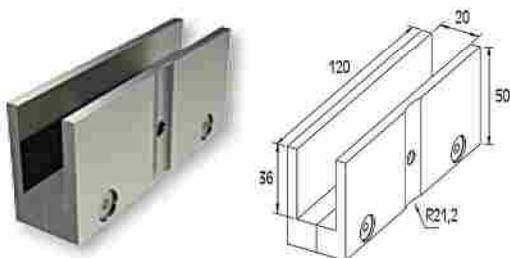
SOPORTE DOBLE CRISTAL 19-22MM PARA COLUMNA DE 42
