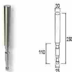
SUJECCIÓN AL SUELO PARA COLUMNA F50-102 Infloor support for F50-102 column
