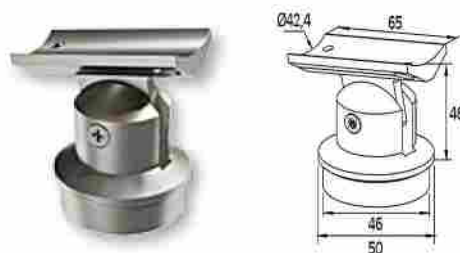
UNIÓN F50-103 CON F50-200 (ESCALERA) Connector for F50-100 column with F50-200 handrail
