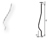
4670 PERFIL CURVADO PARA VERTICAL-D
