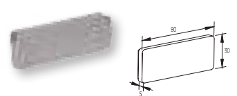
4509 EMBELLECEDOR PASAMANOS
