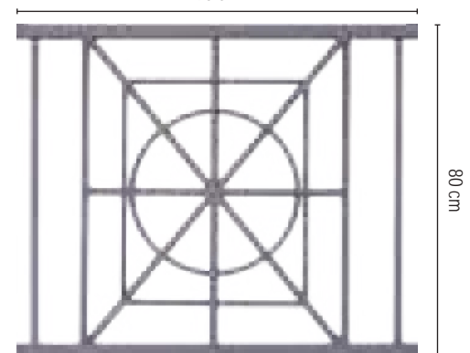
COD. 80 - 21 MOD. GEOMETRICO 96 cm
