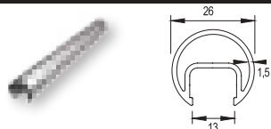
F50-305 RAIL F-26 PARA CRISTAL DE 10 MM.
