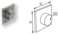
4509A SUJECION PARED A COLUMNA F-200
