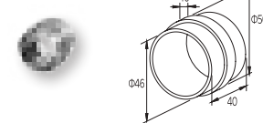
4245 UNIÓN EXTERNA DEL PERFIL F50-102/106 Y PERFIL F50-302
