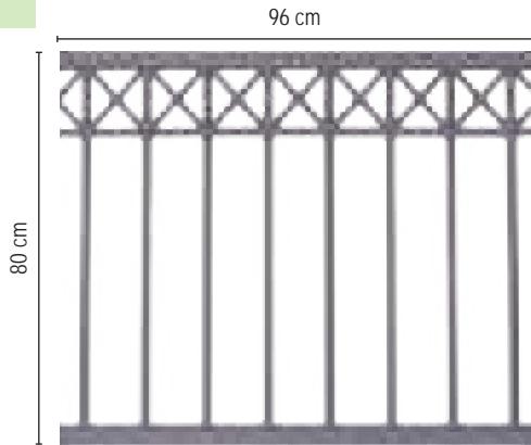
COD. 80 - 01 MOD. INTERNACIONAL 96 cm
