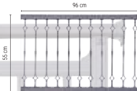
COD. 55 - 16 MOD. ESTRELLA B
