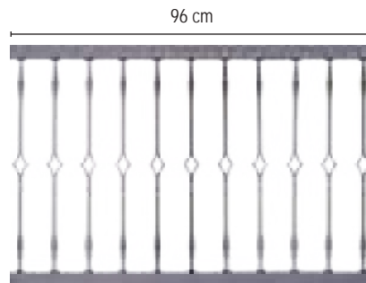
COD. 55 - 17 MOD. ESTRELLA A
