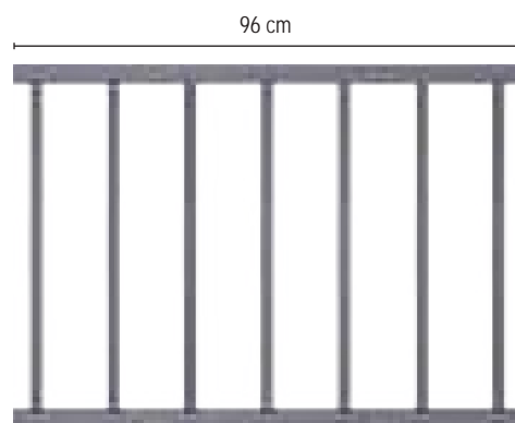
COD. 70-28 MOD. LINEAL SISTEMA LINEAL ABROCHADO El sistema está patentado - N° Patente: 20000200038
