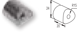
4244 UNIÓN EXTERNA DEL PERFIL F50-102/106 CON F26
