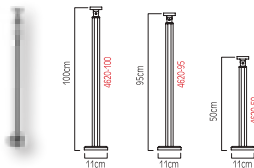
4620 COLUMNA DE SUJECION PREPARADA
