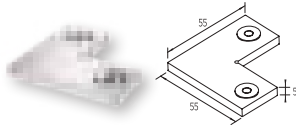
4316 SUJECIÓN PASAMANOS F-50 A COLUMNA F50-100 (ESCALERA)
