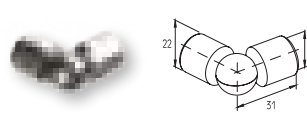
4319 ARTICULACION ESQUINA F-50
