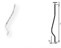
4680 PERFIL CURVADO PARA VERTICAL-D
