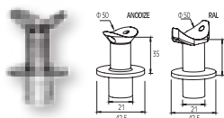
4323 ARTICULACIÓN ESQUINA F-16 CON COLUMNA F50-100
