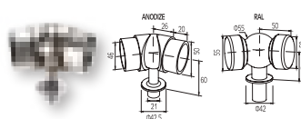
4328 UNIÓN COLUMNA CON PASAMANOS F50-102 CON F50-201
