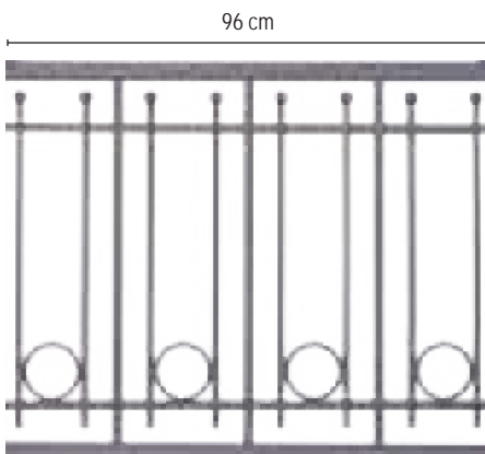
COD. 80 - 22 MOD. KIKLADES 96 cm
