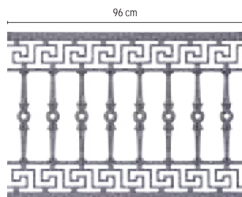
COD. 70-25 MOD. ATENIENSE
