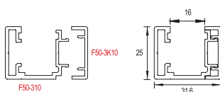
F50-3K10 TAPA EMBELLECEDORA
