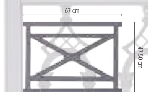
COD. 55-06 MOD. CRISMAS
