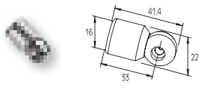
4329 ARTICULACION ESQUINA F-50 PASAMANOS
