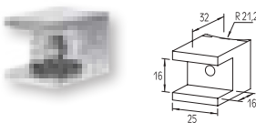
4242 UNIÓN DE RAIL A RAIL
